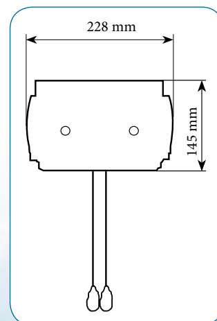
Profile du carter
